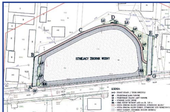
Projekt zagospodarowania przestrzeni w Kaszewskiej Woli.
