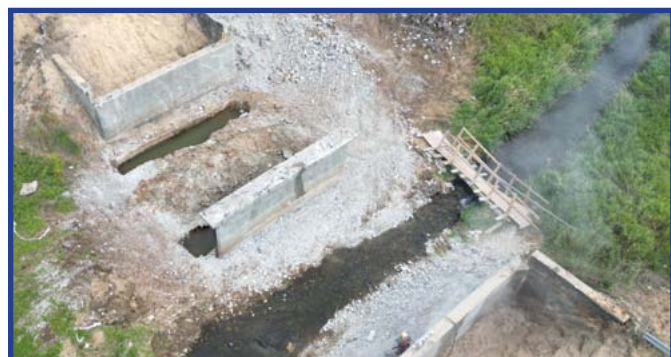
Rozbiórka mostu na rzece Wiązownicy.
