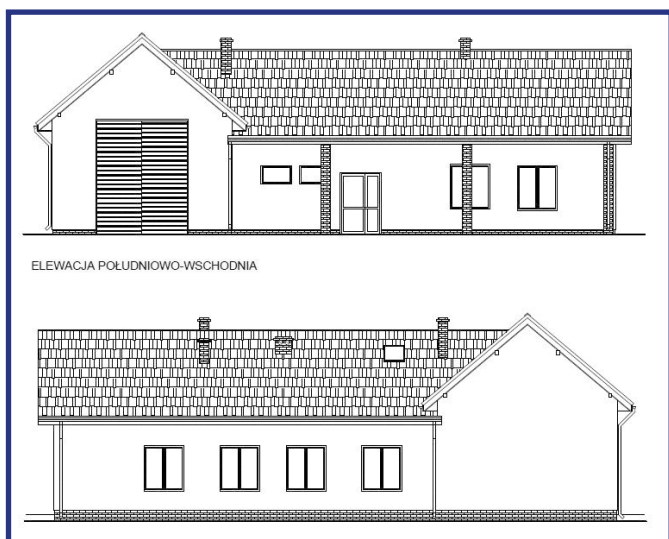
Projekt strażnicy.
